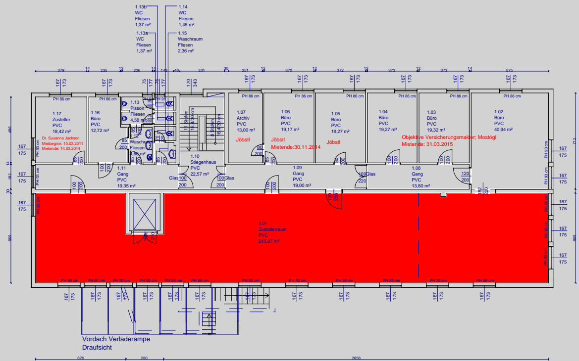
GRUNDRISS 1.OG
