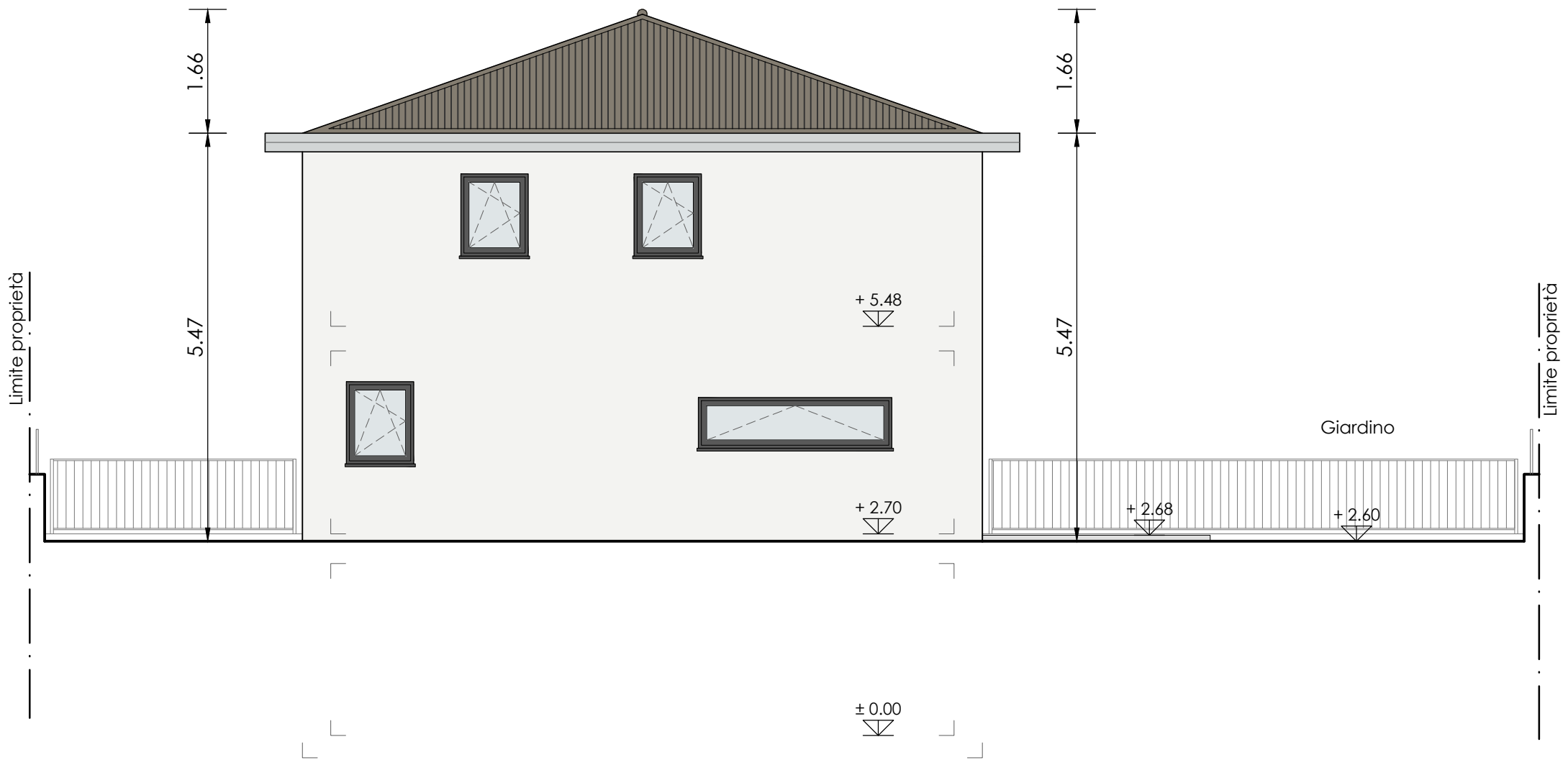
PROSPETTO NORD-OVEST
