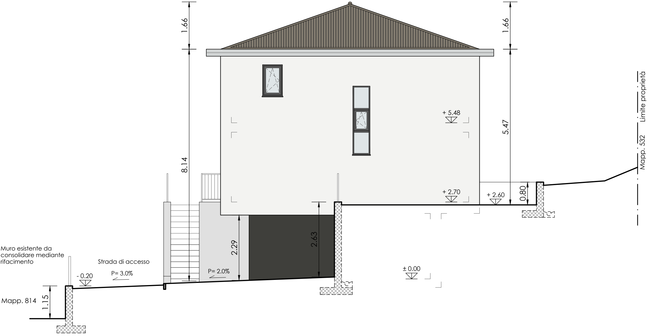
PROSPETTO NORD-EST
