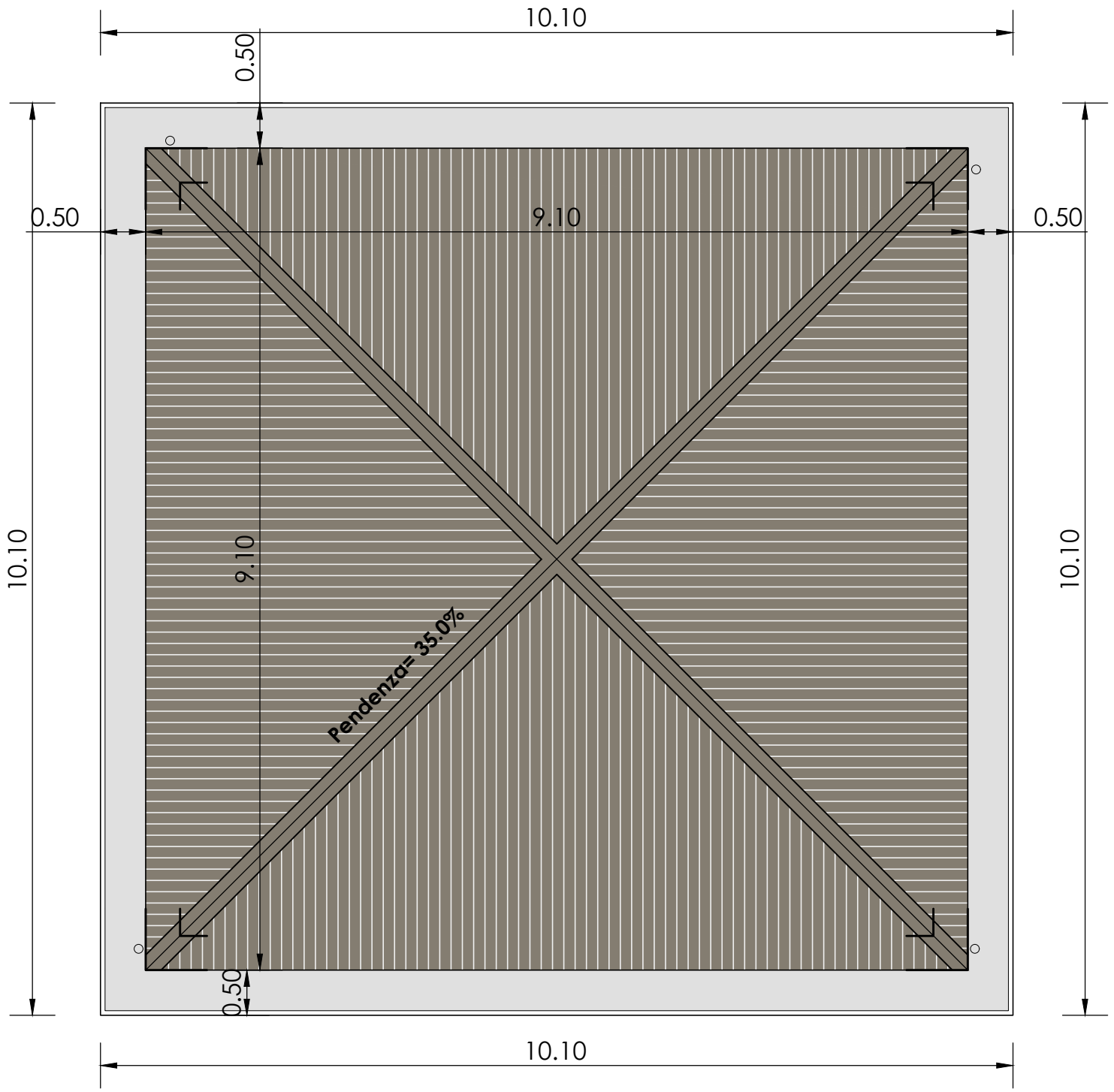
PIANTA DEL TETTO
