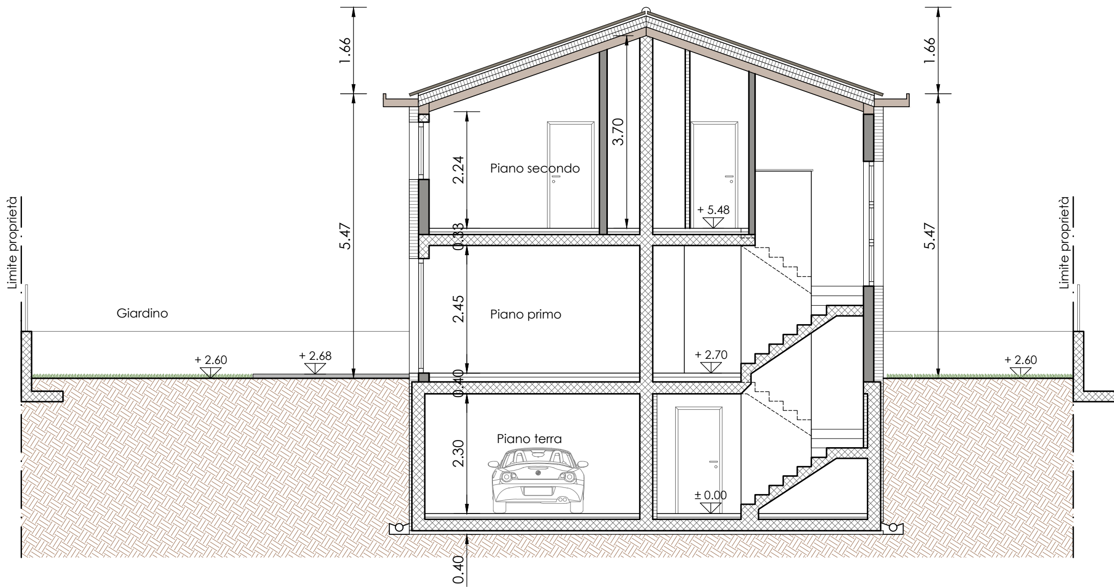
SEZIONE B-B'
