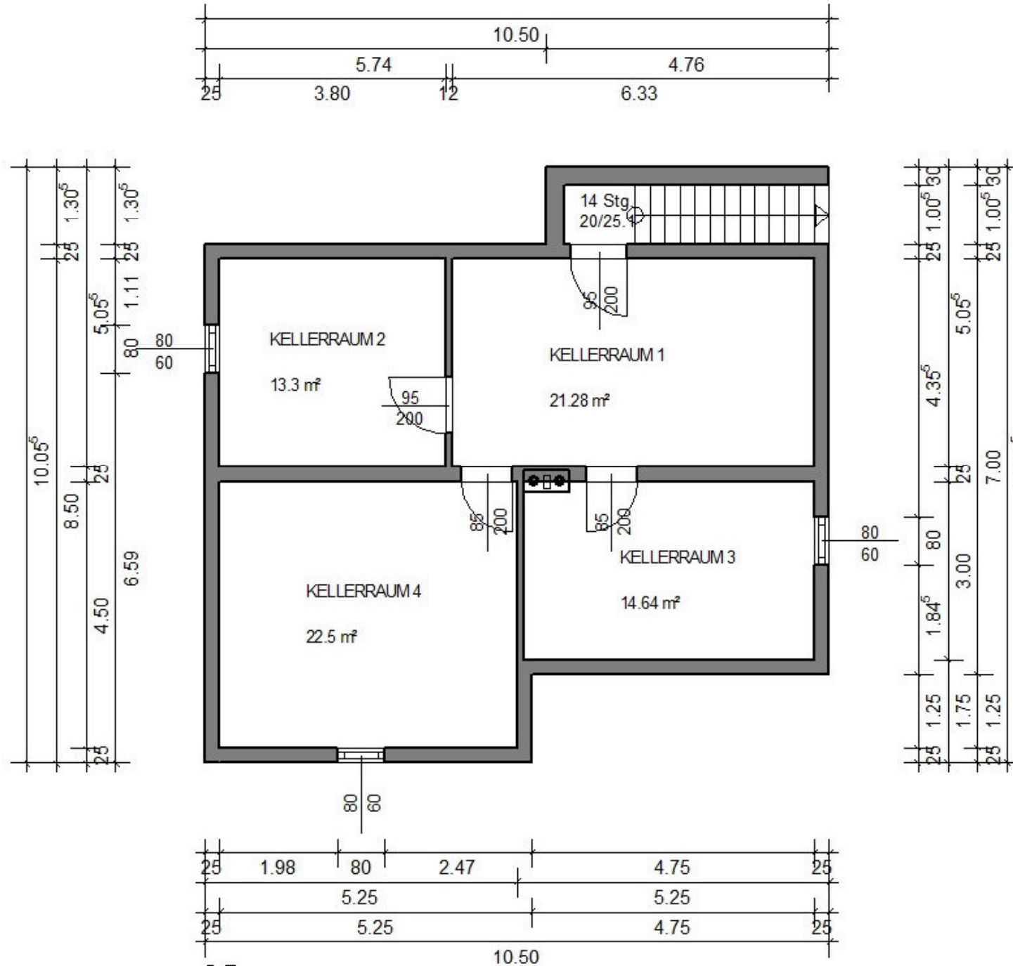
GRUNDRISS KELLERGESCHOSS
