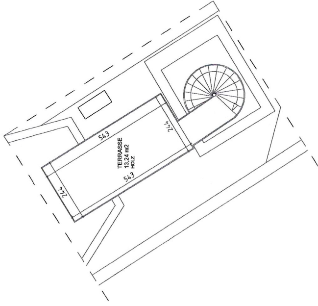
DACHDRAUFSICHT
