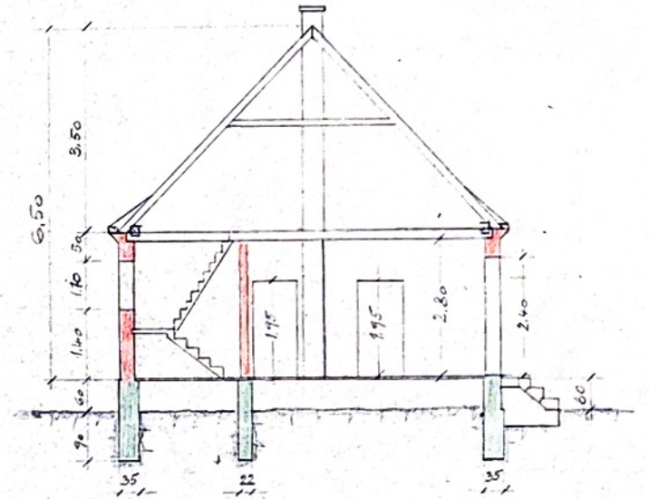
SCHNITT A-A
