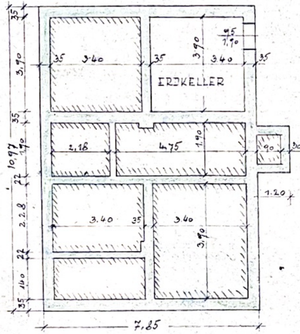
GRUNDRISS
